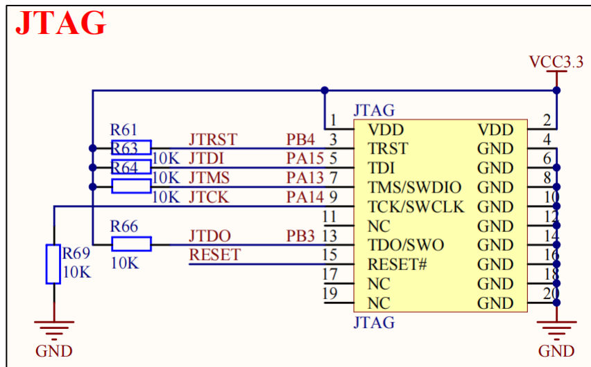
图 2.1.4.1 JTAG/SWD 接口
