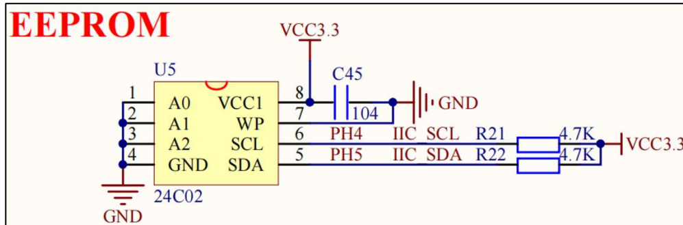
图 2.2.7.1 EEPROM
