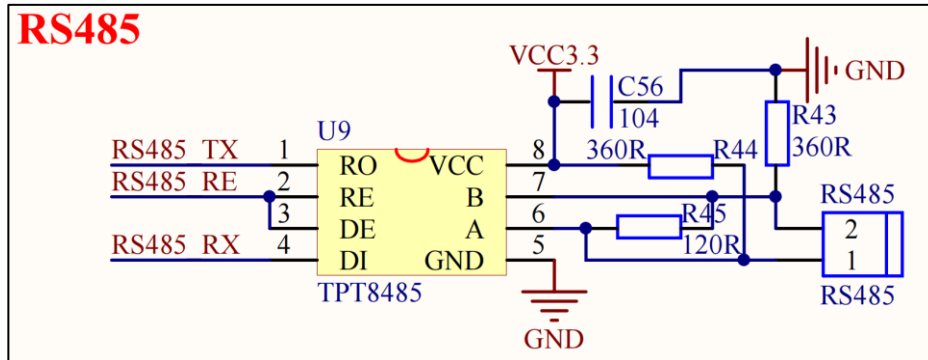
图 2.1.11.1 RS485 接口
