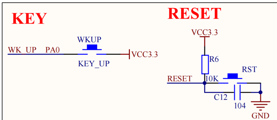
图 2.2.11.1 按键
