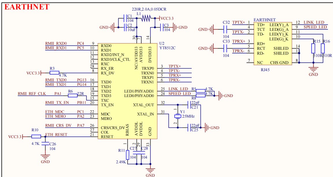
STM32F429 内部自带网络 MAC 控制器，所以只需要外加一个 PHY 芯片，即可实现网络
