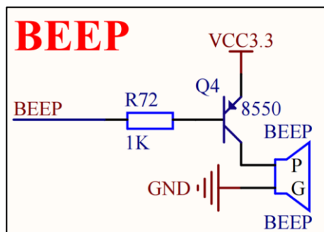
图 2.1.24.1 有源蜂鸣器
