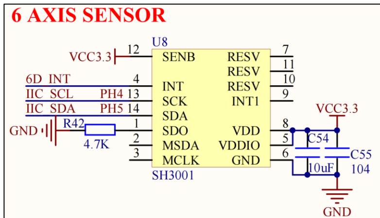
图 2.1.15.1 六轴传感器
