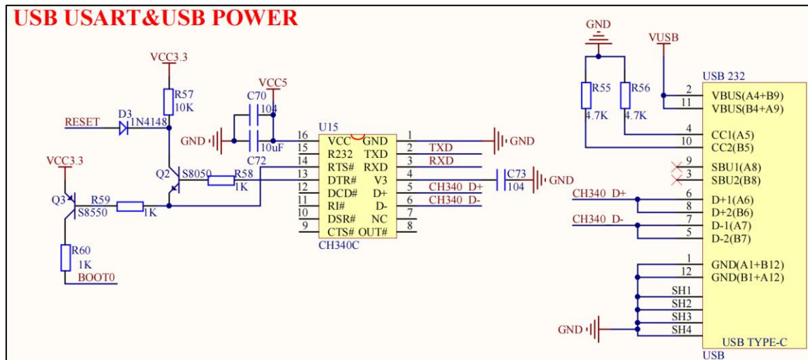
图 2.1.33.1 USB 串口
