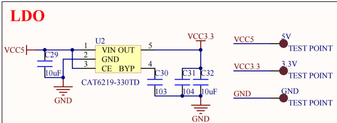
图 2.2.13.1 电源
