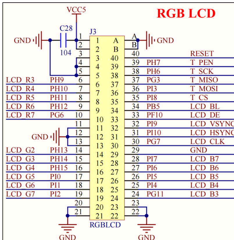
图 2.2.8.1 RGB LCD 接口
