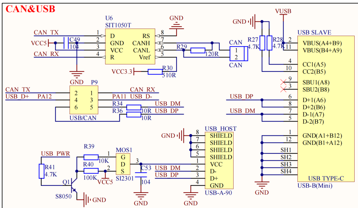
图 2.1.12.1 CAN/USB 接口
