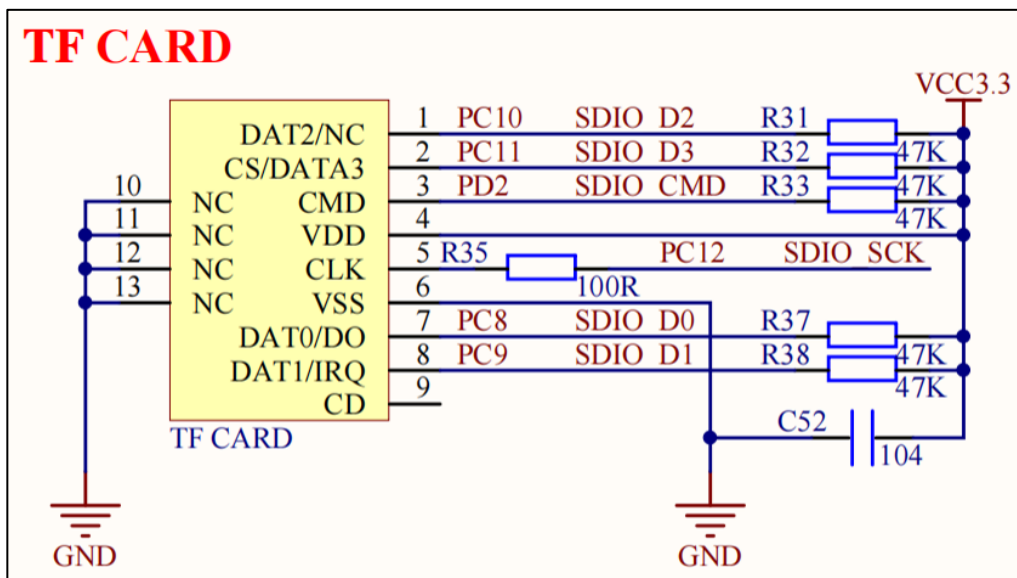
图 2.1.25.1 TF 卡接口
