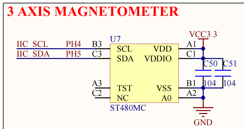
图 2.1.16.1 三轴磁力计
