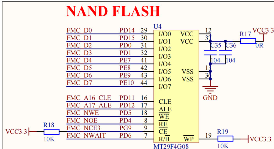
2.2.5.1 NAND FLASH
