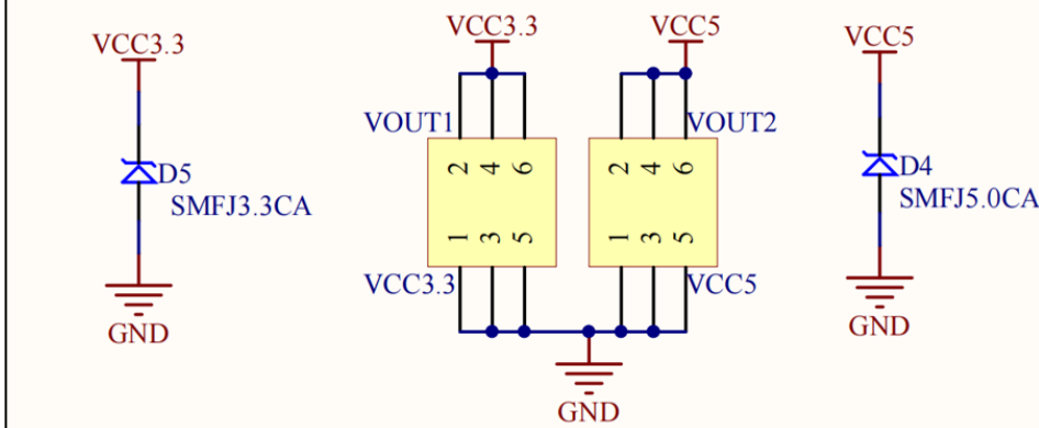
图 2.1.32.1 电源输入输出接口
