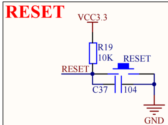
图 2.1.7.1 复位电路
