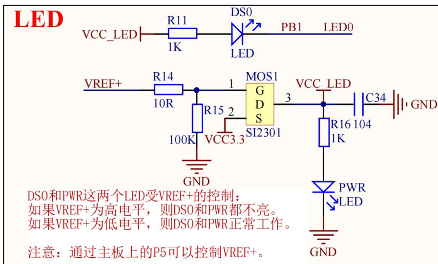
图 2.2.12.1 2 个 LED
