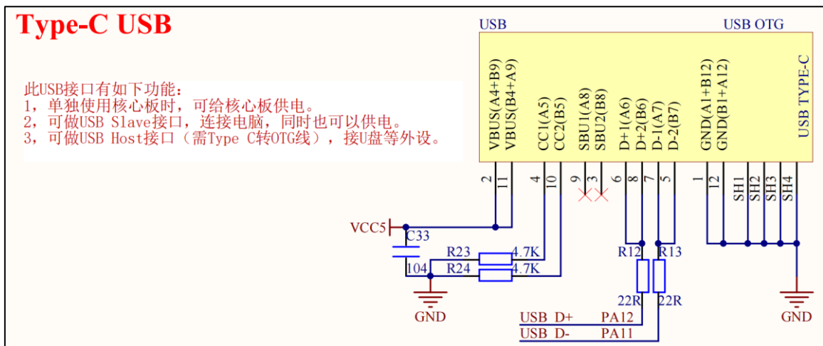
图 2.2.10.1 Type-C USB 接口
