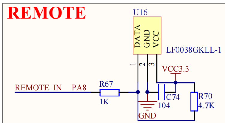
图 2.1.18.1 红外接收头
