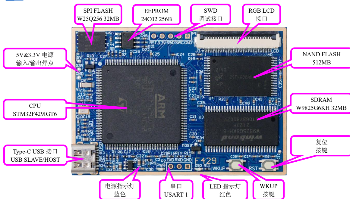
图 1.3.3.1 阿波罗 V2 STM32F429 核心板硬件资源分布图
