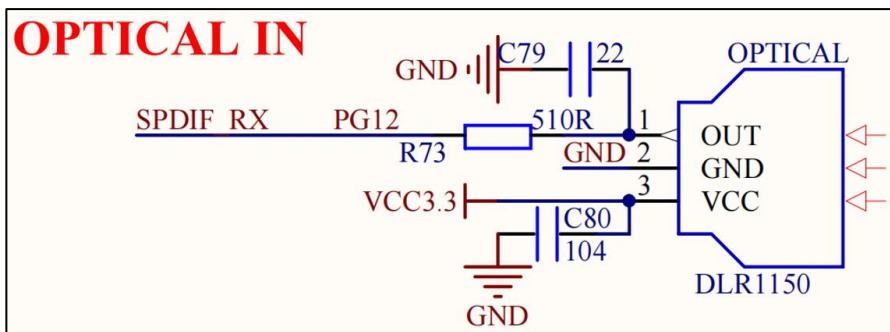
图中，光纤输入采用的是 DLR1150，输出信号经过 SPDIF_RX 传输给 MCU，SPDIF_RX 连接在 MCU 的 PG12 上面。SPDIF_RX 和 NRF_CE 共用 PG12，所以光纤接口和无线模块接口，不可以同时使用，不过，可以分时复用。 特别注意：对于 STM32F429，这个接口是没有用的，只有 STM32F767/H743 才有 SPDIF 接收功能，才可以使用此接口。
